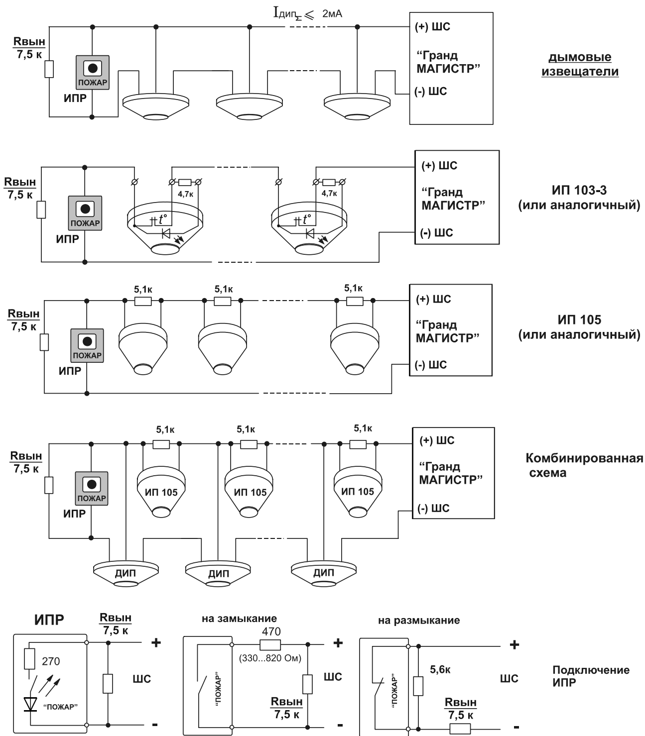
Рис. 7. Организация однопорогового шлейфа пожарной сигнализации
