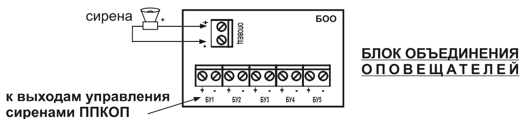
Рис. 10.2. Схема подключения одного звукового оповещателя (сирены) к нескольким приборам "Гранд МАГИСТР"
