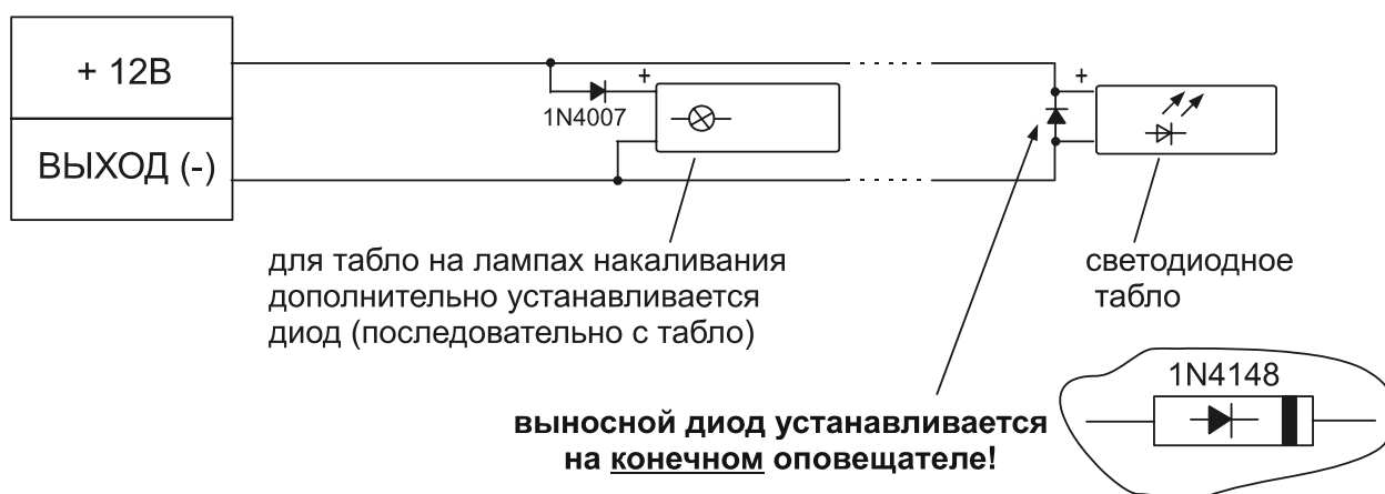
Рис. 9. Схема подключения нескольких световых табло
