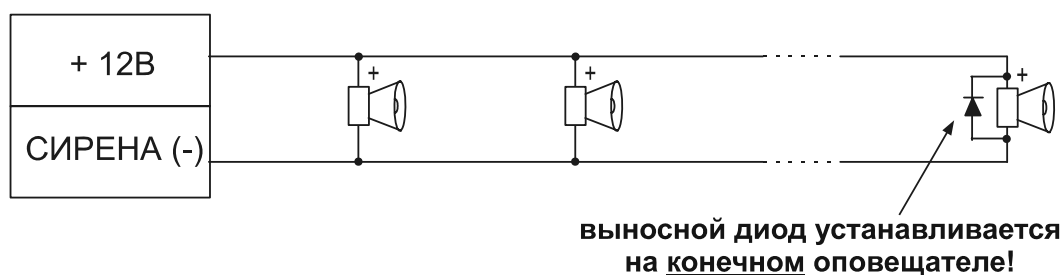
Рис. 10.1. Схема подключения нескольких звуковых оповещателей
