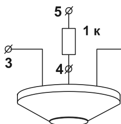
Рис. 5. Организация двухпорогового шлейфа пожарной сигнализации
