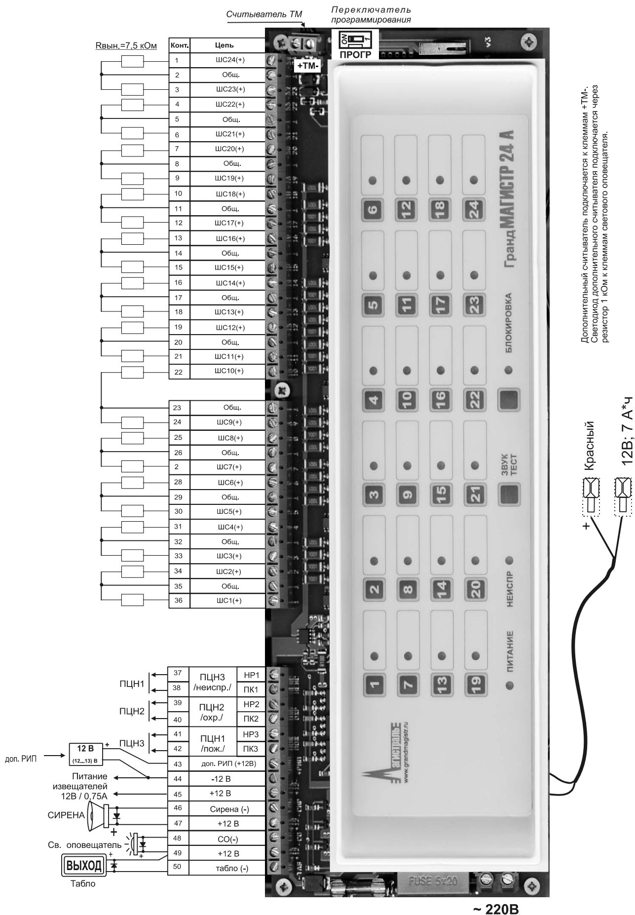
Рис 4. Схема внешних соединений прибора "Гранд МАГИСТР" исполнений -12А, -16А, -20А, -24А
